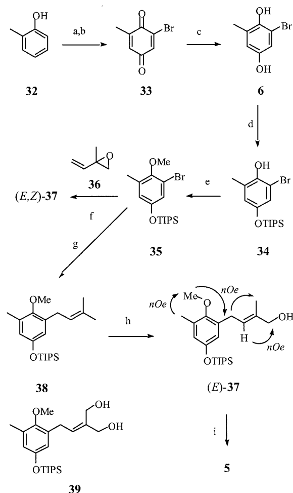
Scheme 6. Synthesis of the aromatic subunit 5 : a) Br 2 , AcOH, 20 °C, 96%; b) CrO 3 , AcOH, 0 °C, 5 h, 95%; c) Na 2 S 2 O 4 , EtOH, 20 °C, 2 h, 52%; d) TIPSCl, Imidazole, DMF, 18 h; e) CH 3 I, K 2 CO 3 , acetone, reflux, 4 h, 70% from 6 ; f) i : n BuLi, Et 2 O, −78 °C ii : CuCN, LiCl, −30 °C, 30 min iii : 36 , −78 °C to 20 °C, 1 h, 67%; g) i : PhLi, Et 2 O, 0 °C, ii : BrCH 2 CH=C(CH 3 ) 2 , DMPU, 20 °C, 18 h, 91%; h) i : SeO 2 , dioxane, water, 100 °C, 1 h, ii : NaBH 4 , EtOH, 15 min, 20 °C, 60%; i) Br 2 , Ph 2 PCH 2 CH 2 PPh 2 , CH 2 Cl 2 , 20 °C, 2 h, 88%
